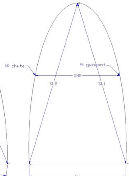
SPI SYMETRIQUE
